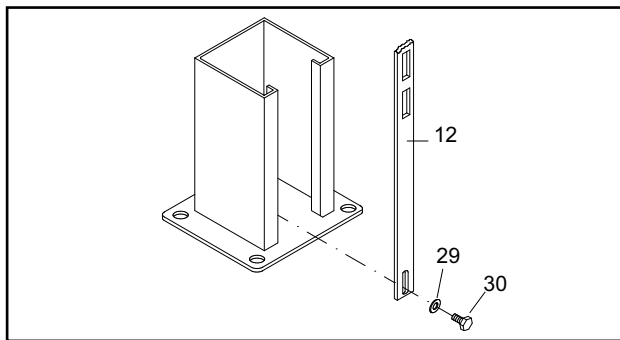
Fig.47 Bloccaggio dell'asta di sicurezza Fig.47 Safety rod locking
