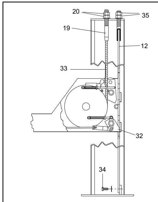
Fig.54 Preregistrazione funi
