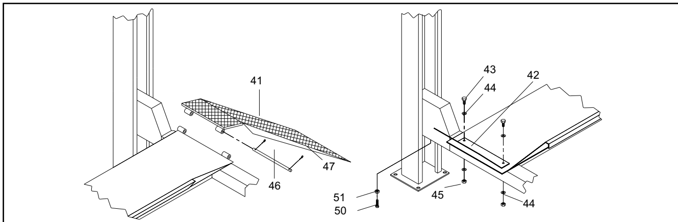
Fig.59 Fissaggio rampe e bloccaggi ruote
