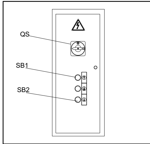
Fig.53 Pannello di controllo
