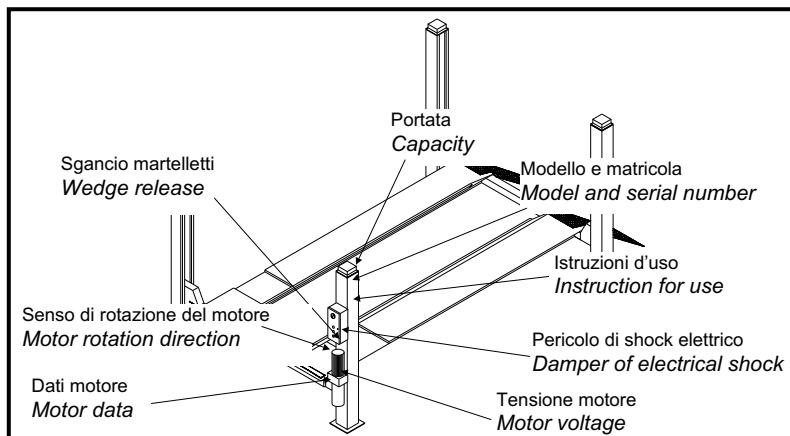
Fig.37 Avvisi di sicurezza e targhette applicati sulla macchina
