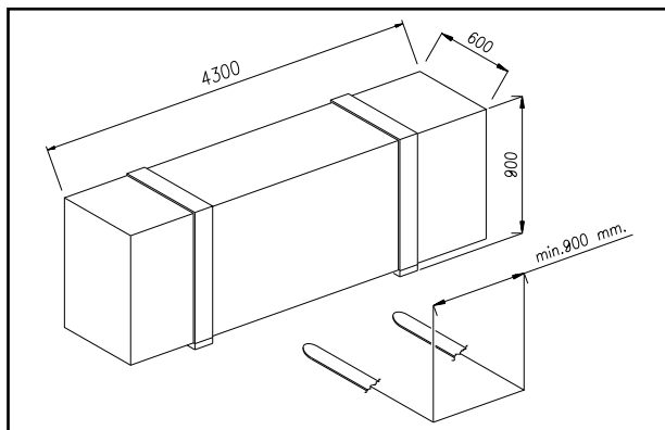
Fig.1 Imballo e spostamento - Packing and moving
