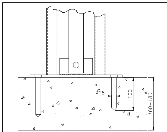
Fig.58 Fissaggio delle colonne
