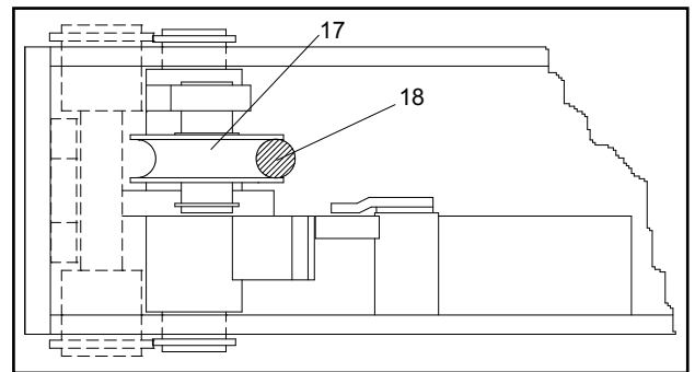
Fig.48 Posizionamento dei sensori fune Fig.48 Positioning of lifting cable sensors
