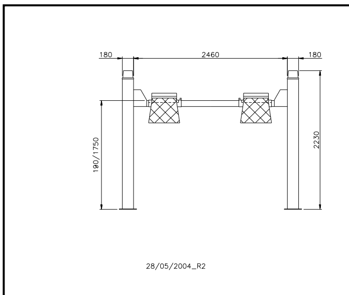
Fig.11a - Dimensioni ed ingombri con pedane senza incavo per assetto ruote
