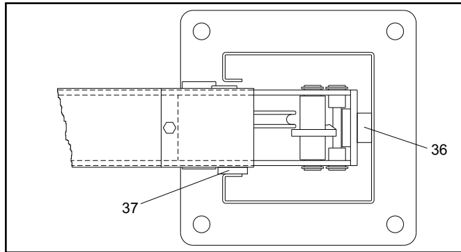
Fig.56 Regolazione pattini
