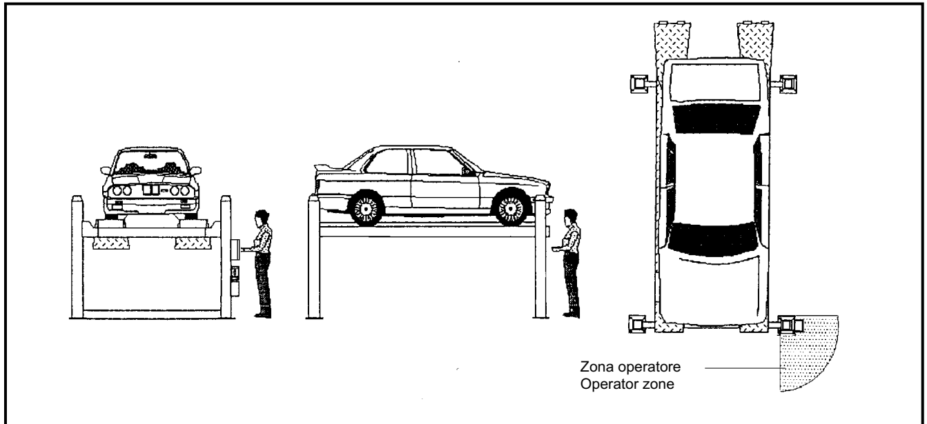
Fig.28 Zona riservata all'operatore
