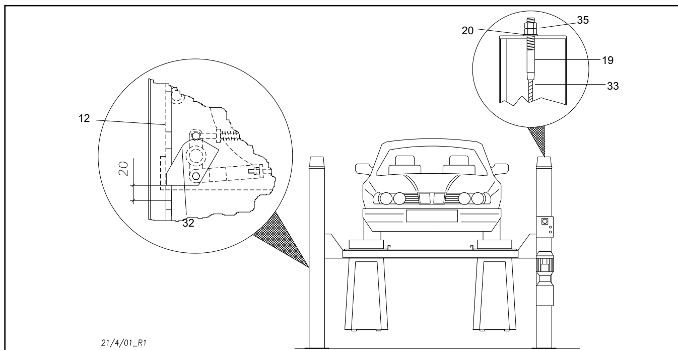
Fig.60 Registrazione funi
