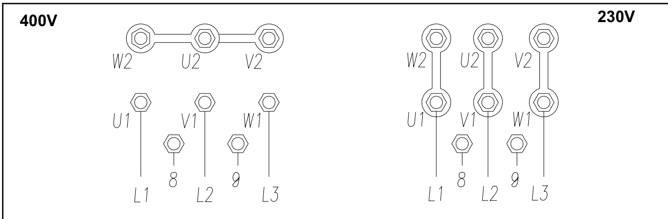
Fig.51 collegamenti motore e trasformatore
