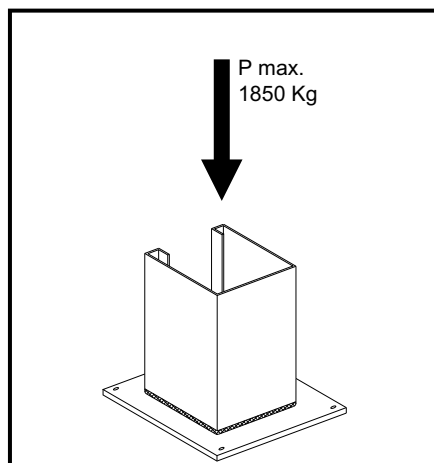
Fig.39 Carichi sulle fondazioni
