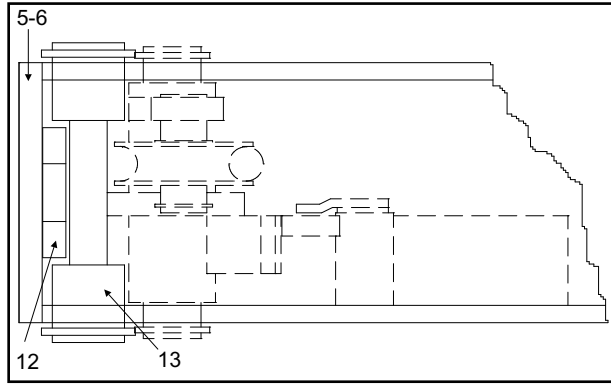
Fig.46 Sede di inserimento dell'asta di sicurezza
