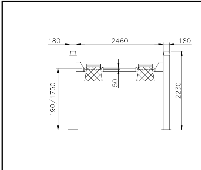
Fig.11 - Dimensioni ed ingombri con pedane per assetto ruote
