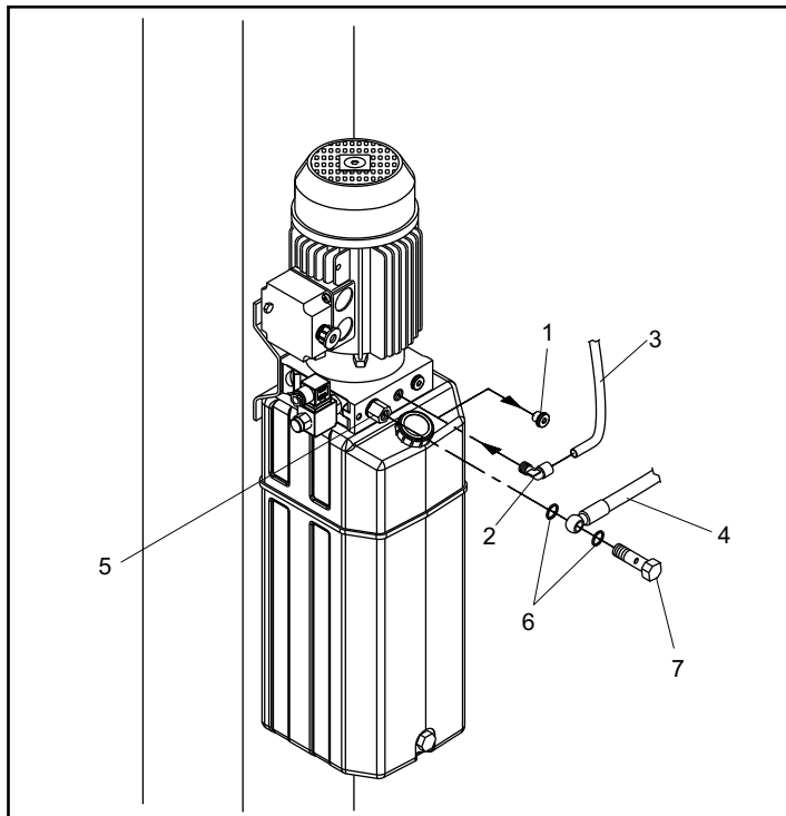
Fig.49Allacciamento impianto idraulico Fig.49Hydraulic system connection
